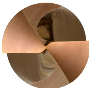
Kąty wierzchołkowe 120°, 145°
