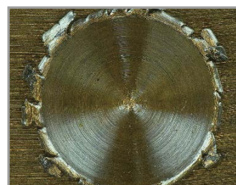
Wiertło konwencjonalne
